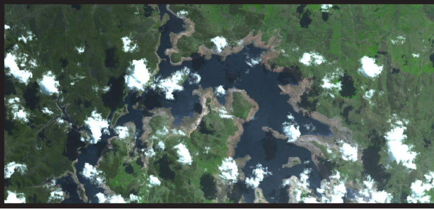
Satelliittikuva kuivuuden pienentämästä Eucumbene-järvestä Australiassa
