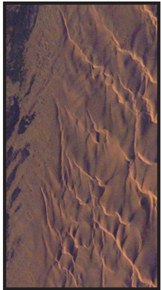
Dyynikuvioita Namibin autiomaassa Namibiassa avaruudesta kuvattuna (kuva: Nasa, www.nasa.gov )
